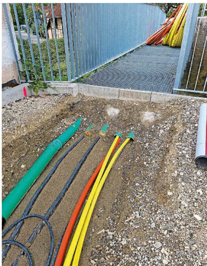
Verlegte Breitbandpipe im Bereich der Brücke Fotos: Stadt Tengen
